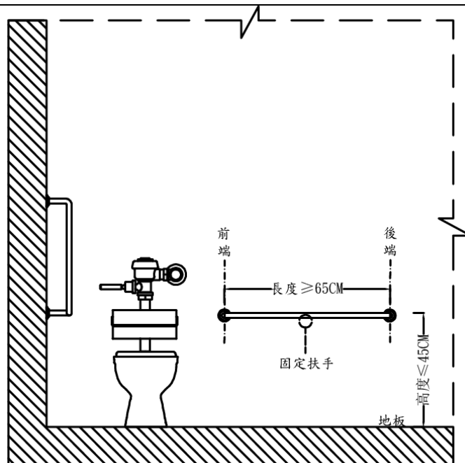
圖2-4 (固定扶手)
