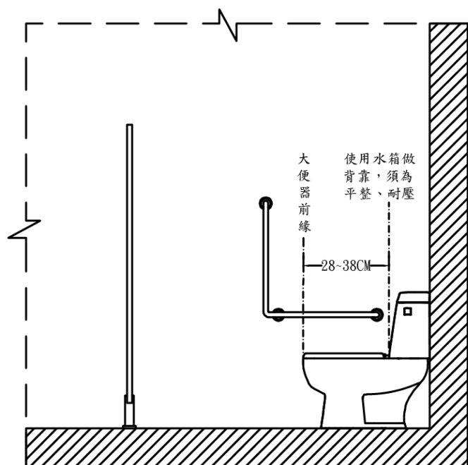
圖2-5 (背靠)
