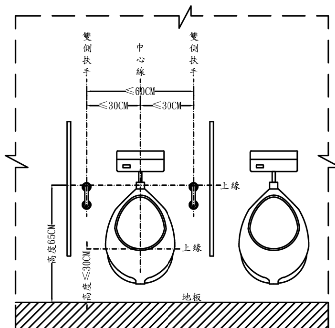
圖3-2（扶手上緣距地板面距離）
