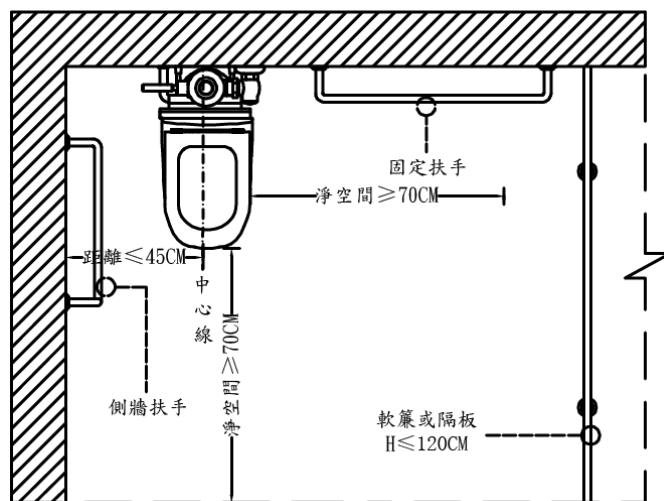
圖2-1(側邊淨空間)
