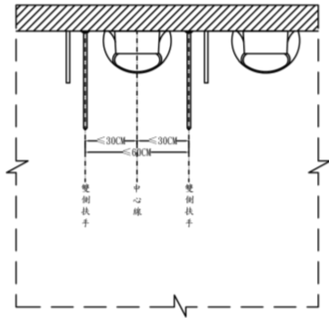
圖3-1（雙側扶手距離）
