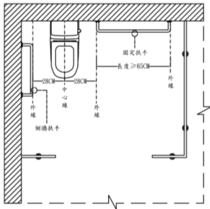
圖2-3 (扶手外緣與大便器中心線距離)
