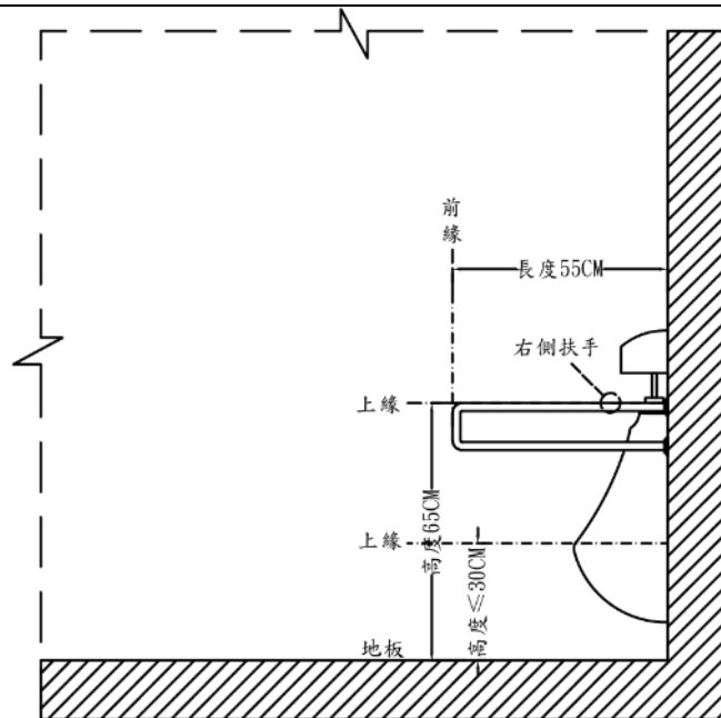
圖3-3 (雙側扶手長度)
