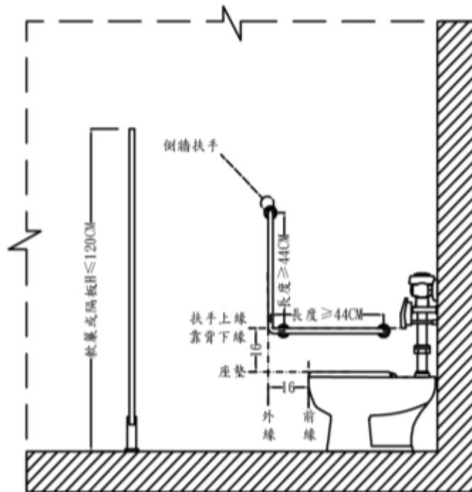
圖2-2(側邊 L 型扶手)
