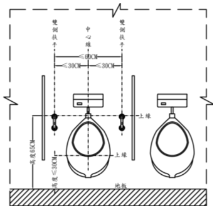
圖3-2（扶手上緣距地板面距離）
