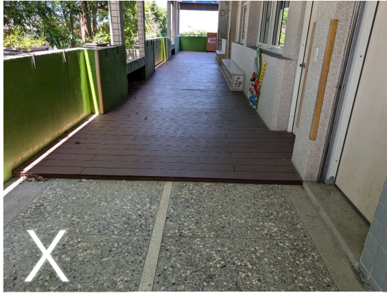
高差在0.5公分至3公分者，應作1/2之斜角處理
