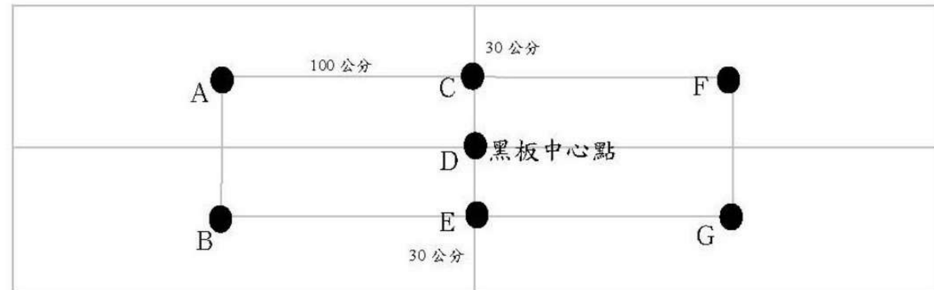
圖 7 黑板面照度檢測點
